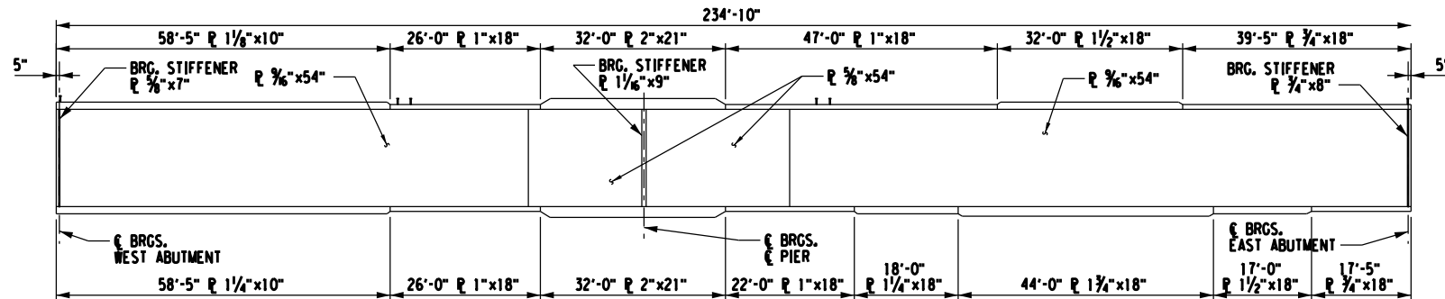
GIRDER ELEVATION N.T.S.
