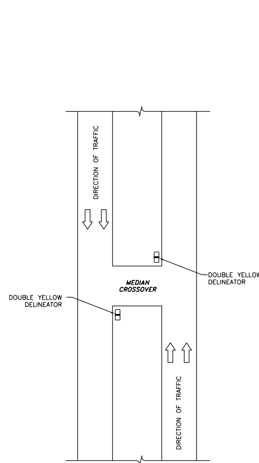
DELINEATOR LAYOUT MEDIAN CROSSEOVERS N.T.S.
