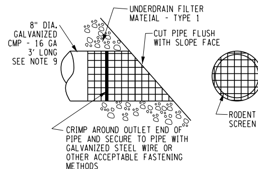
PIPE END - DETAIL A N.T.S.
