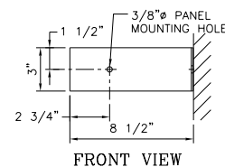
WALL MOUNT BRACKET N.T.S.
